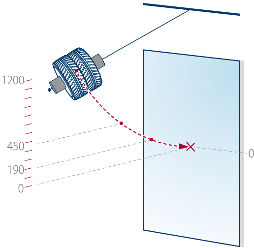
The pressure of the tyres: p - (0,35 \pm 0,02) \text{ MPa}
